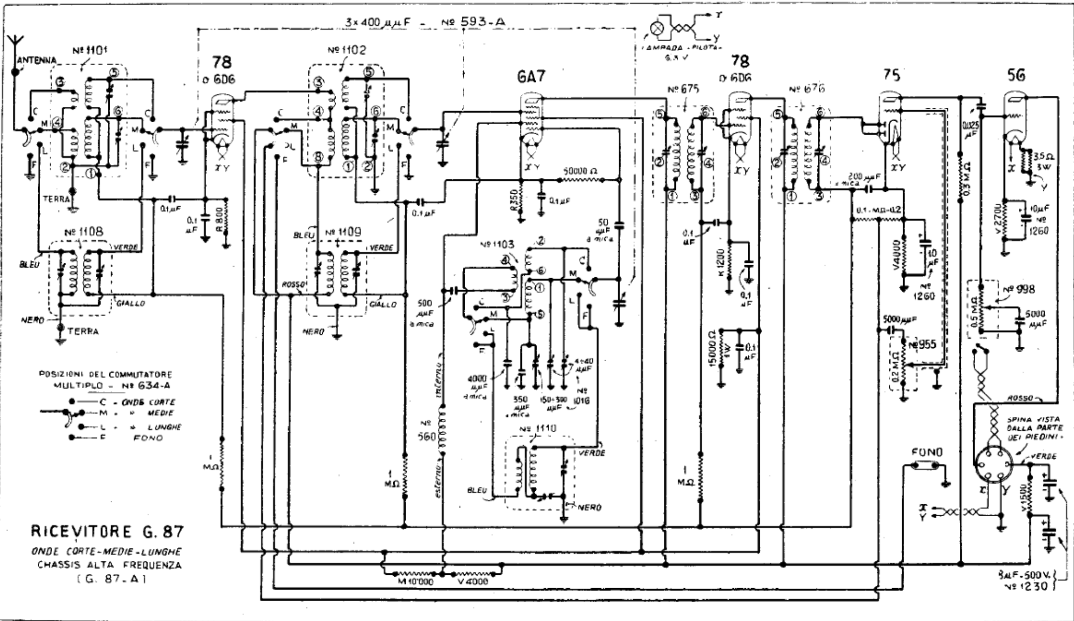
- Schema elettrico del ricevitore (Chassis A.F.).
